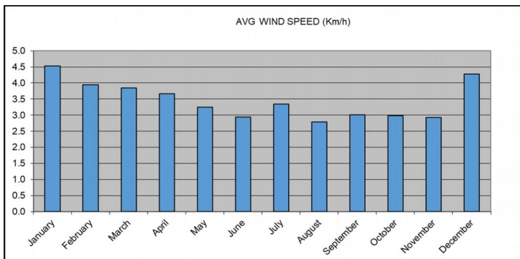
Γράφημα 10: Μηνιαία διακύμανση της μέσης ταχύτητας ανέμου (Km/h) για το σταθμό Ζαγοράς Πηλίου (Πηγή: ΠεΣΠΚΑ, 2020)
