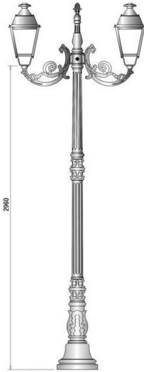
Φωτ. 5: Ενδεικτικό φωτιστικό σώμα, παραδοσιακού τύπου φανάρι, διπλό
